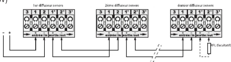
SCHEMA DE RACCORDEMENT
