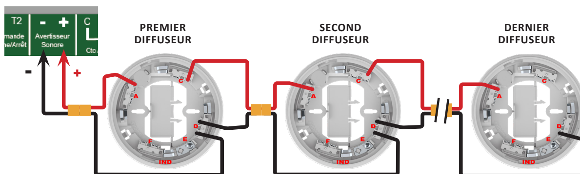
2 boucles 11225
