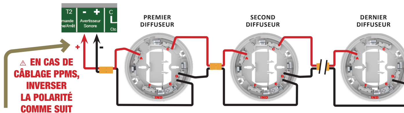
Câblage PPMS
